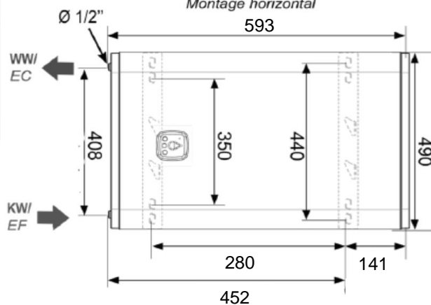
Horizontale Montage / Montage horizontale
