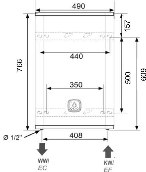
Horizontale Montage / Montage horizontale
