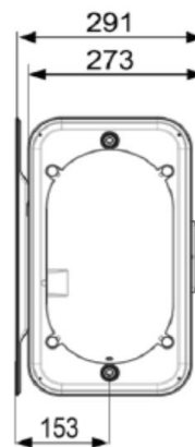
Unterseitensicht / Vue de dessous
