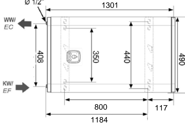
Horizontale Montage / Montage horizontale
