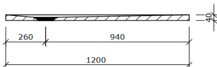
Schnitt A-A (1 : 15)
