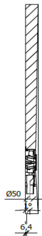
Schnitt B-B (1 : 15)
