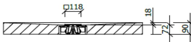
Schnitt A-A (1 : 15)
