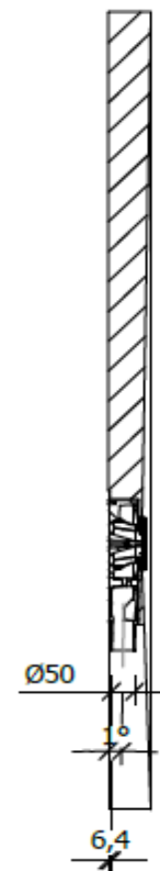
Schnitt B-B (1 : 15)
