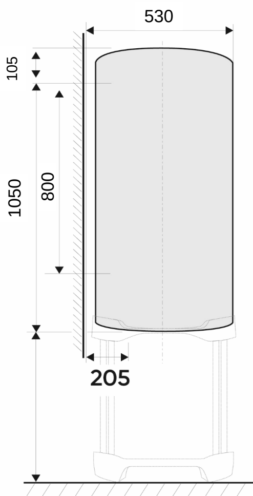
Montage mit einem Auflagegestell Montage avec trépied
