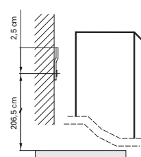
Montageschiene Support de montage Stecca di montaggio
