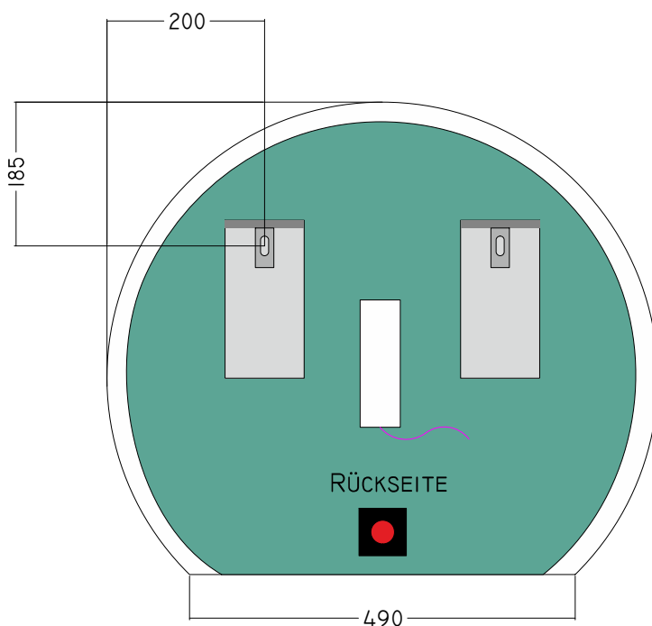
RÜCKANSICHT
