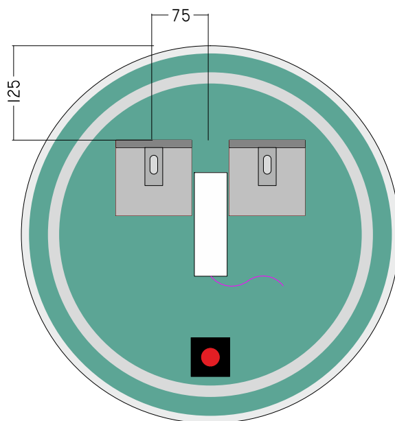
RÜCKANSICHT
