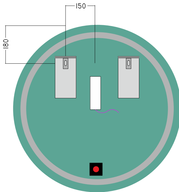
RÜCKANSICHT
