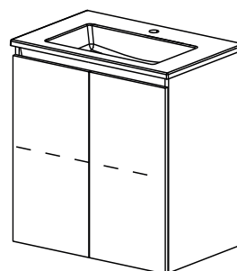
Decoupe pour siphon réduit Ausschnitt für Raumspar-siphon
