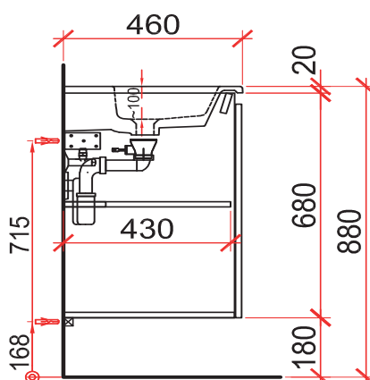
Decoupe pour siphon réduit Ausschnitt für Raumspar-siphon
