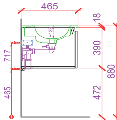
Decoupe pour siphon réduit Ausschnitt für Raumspar-siphon
