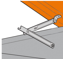
3212 - Hochstellschere kpl. Nachruest- satz
