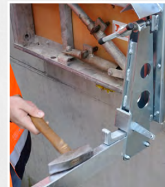
Schlittenkeil mit Hammer anschlagen
