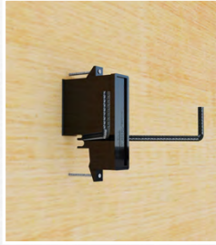
Aussparung aufsetzen ggf. mit Nägeln sichern
