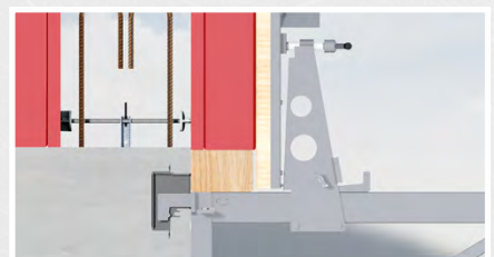
Höchste Sicherheit und freie Auflagefläche
