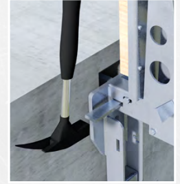
Mit Keil festziehen
