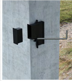
Nach dem Betonieren Zapfen entfernen
