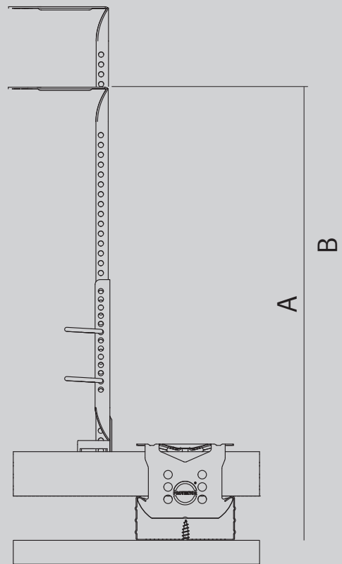
Minimale (A) und maximale (B) Abhänghöhe
