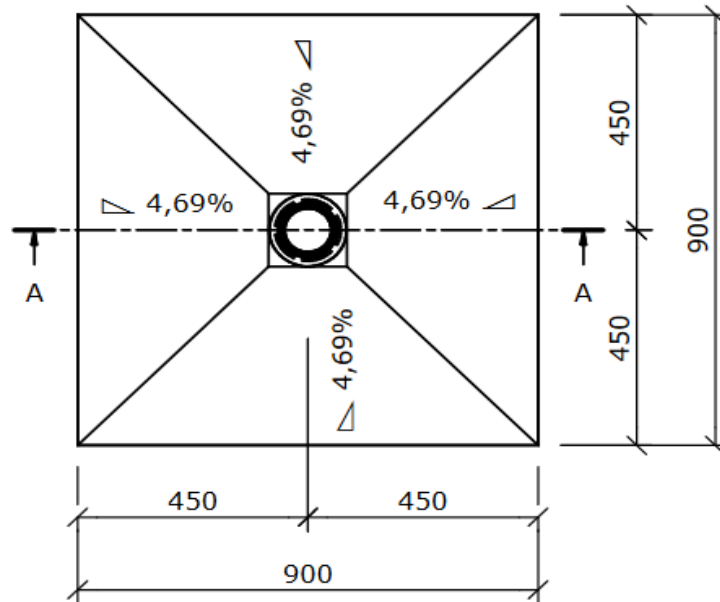
Draufsicht ( 1 : 15 )
