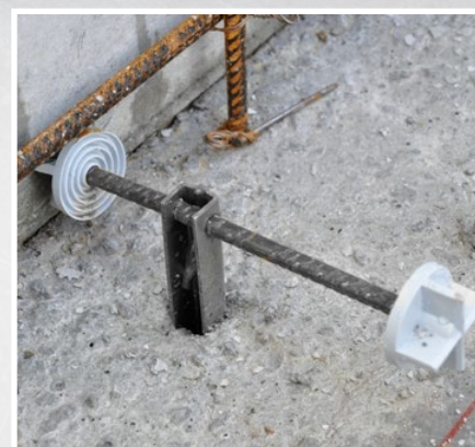
AHB Anschlaghalterung
