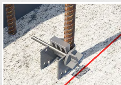
UNO MAX XL 7.5 für Anschlussseisen Ø 22-40 mm
