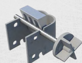
Artikel 2495 UNO MAX XL 7.5 für Anschlusseisen Ø 22-40 mm
