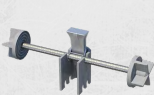
Artikel 2425 UNO MAX 25 cm für Anschlusseisen Ø 6-20 mm
